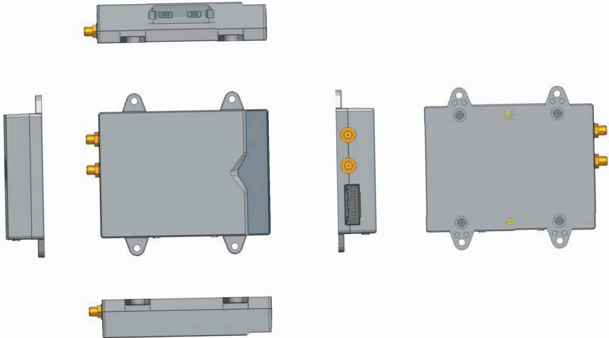
M100 GNSS 接收机-六视图
